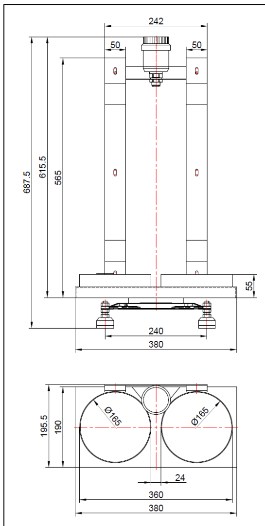
PT500-110-02 型
