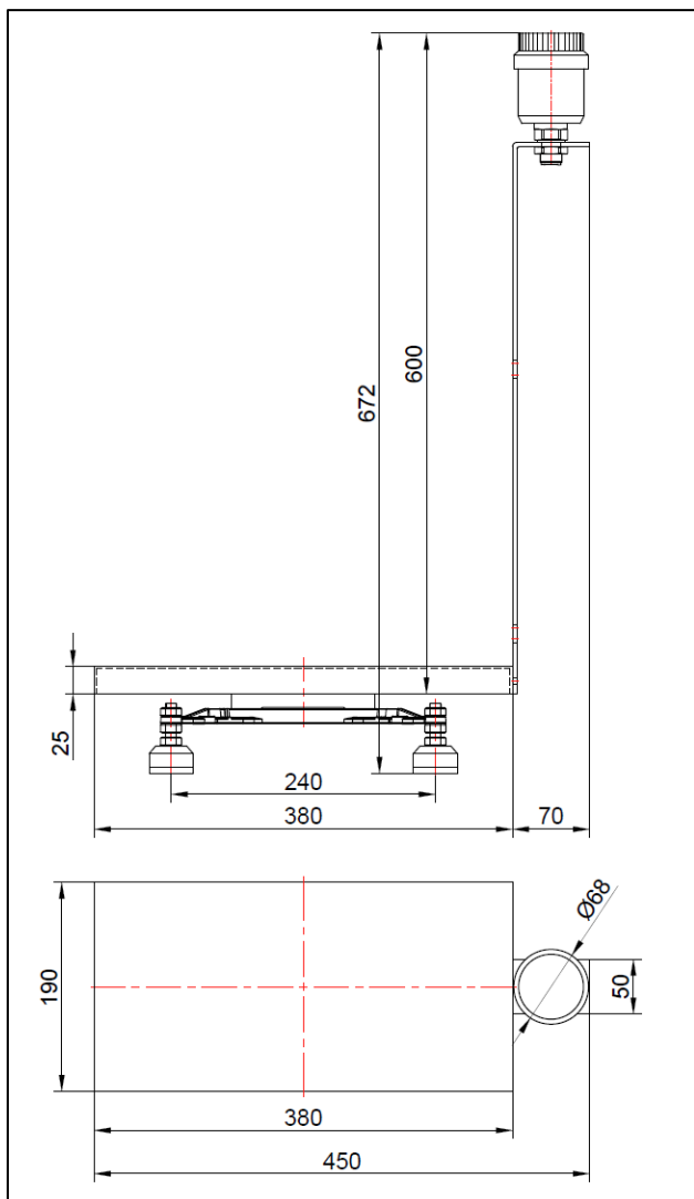
PT500-110-03 型
